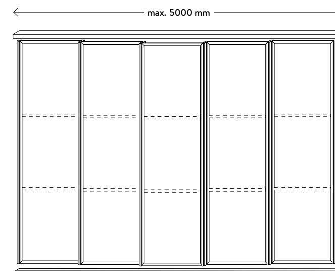
GSSET-011 3-läufiges Gleittürsystem mit 5 Türen
