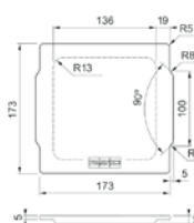
Buchenholz Verschlussdeckel
