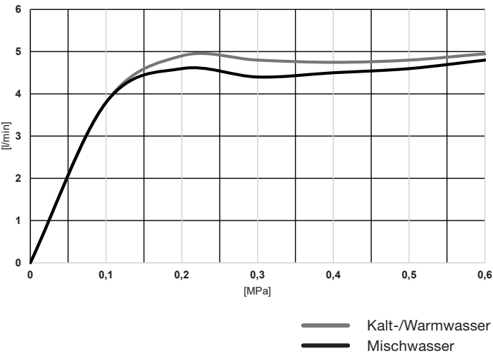
Durchflussdiagramm BLANCO MILA ECO RH HP CHR
