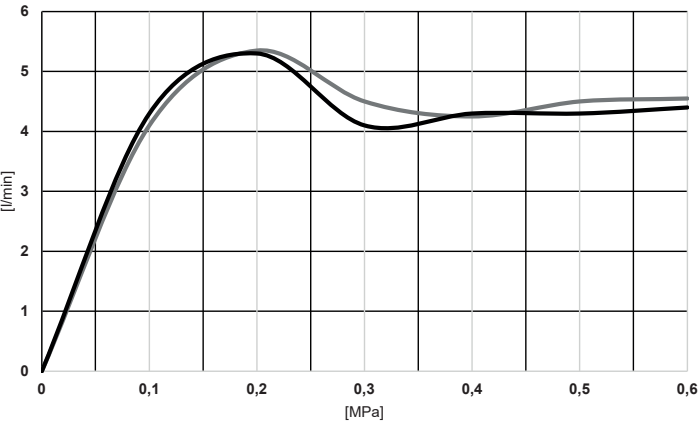
Durchflussdiagramm BLANCO LANORA ECO RH HP BF
