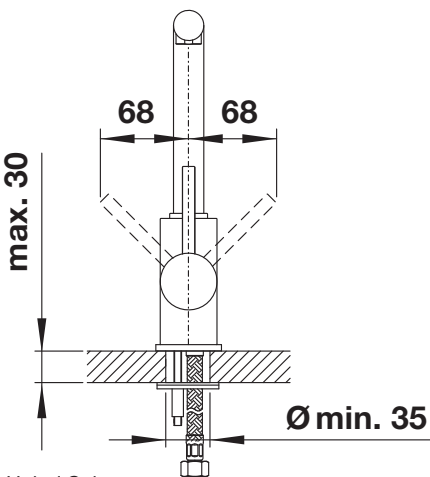
Hebel Seitenansicht
