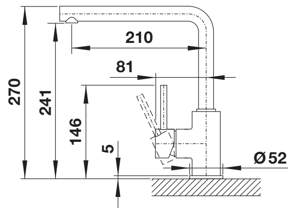
Seitenansicht
