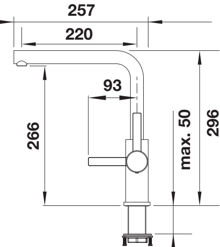
Seitenansicht
